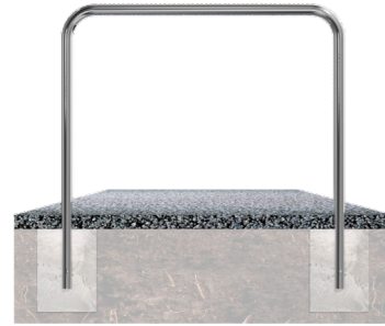
ohne Querholm, zum Einbetonieren
